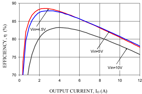
Vo=0.69V
