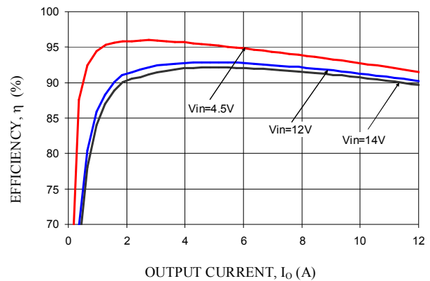
Vo=2.5V
