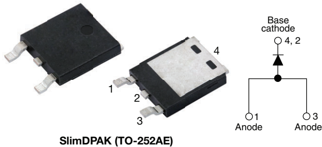
SlimDPAK (TO-252AE)
