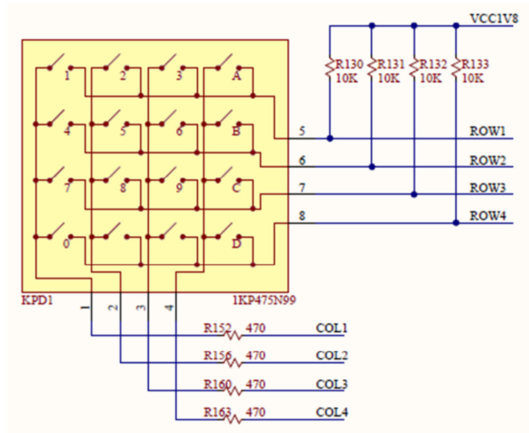
Fig. 13. Keypad schematic
