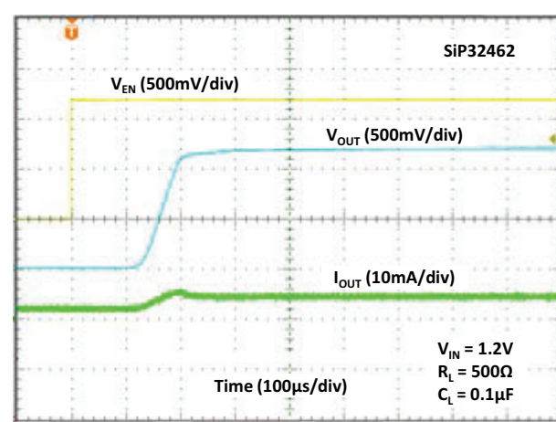
Fig. 30 - Turn-on Time
