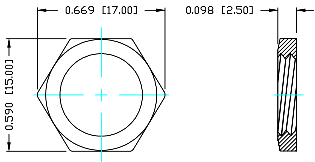
NUT
