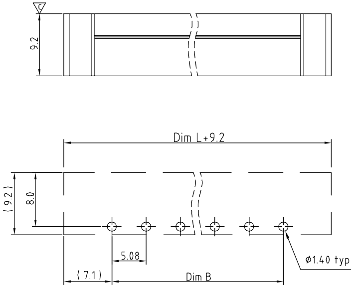
P.C.B Layout
