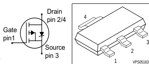
PG-SOT223
