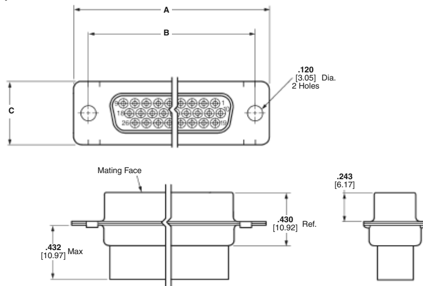
Receptacle
