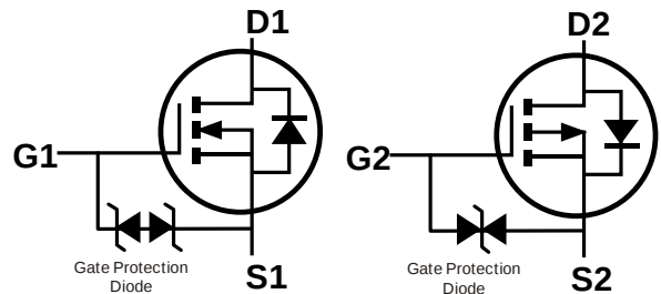
Q1 N-Channel
