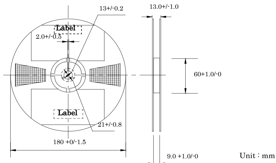
Reel Dimensions
