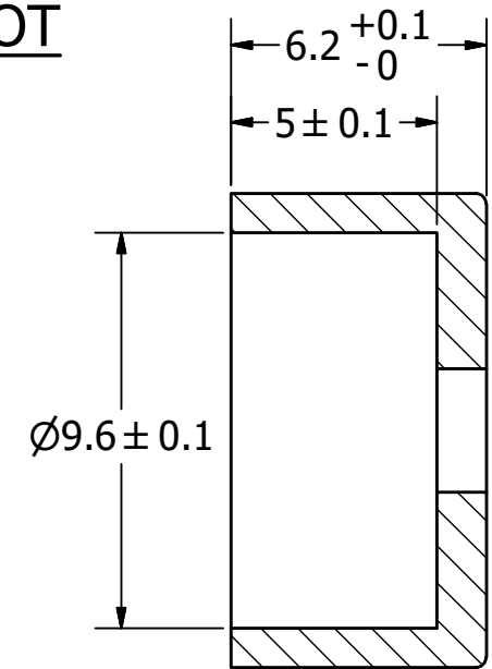
A-A ( 5 : 1 )
