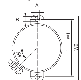
Code J (2—legs)
