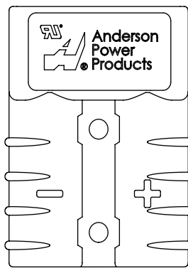
SB®50
