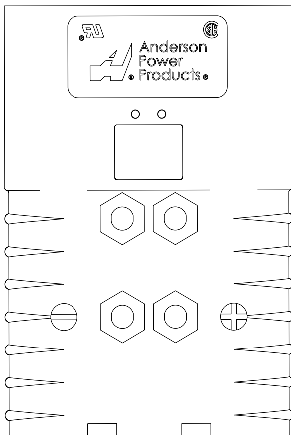
SBE®320 - SBX®350
