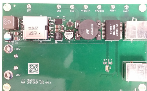
Bottom Side
