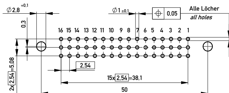
Leiterplatten-Lochbild / PCB drillhole pattern
