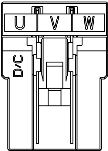
3POS(X-KEY): 1-2013522-3
