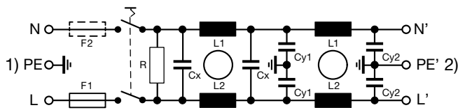
1) Line 2) Load
