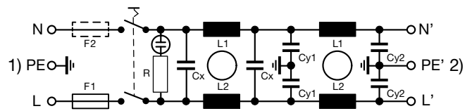
1) Line 2) Load
