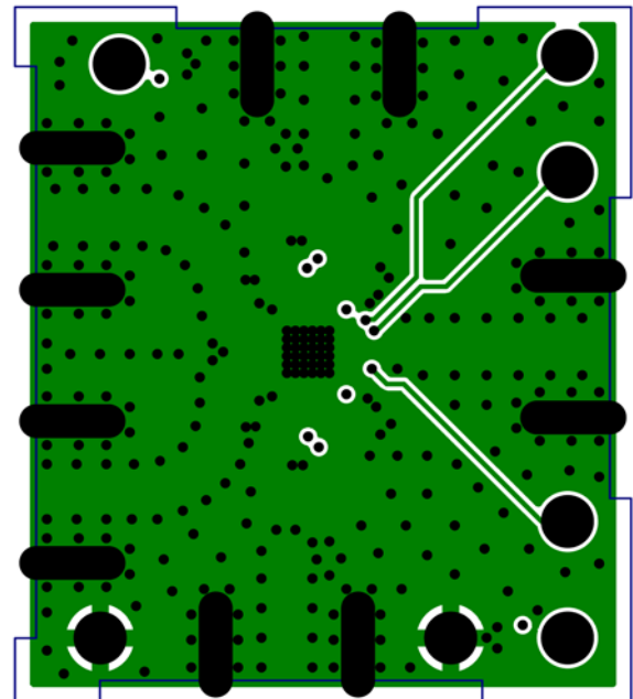
Layer 4. Bottom Layer
