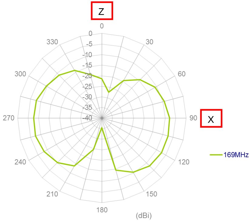
XZ-Plane
