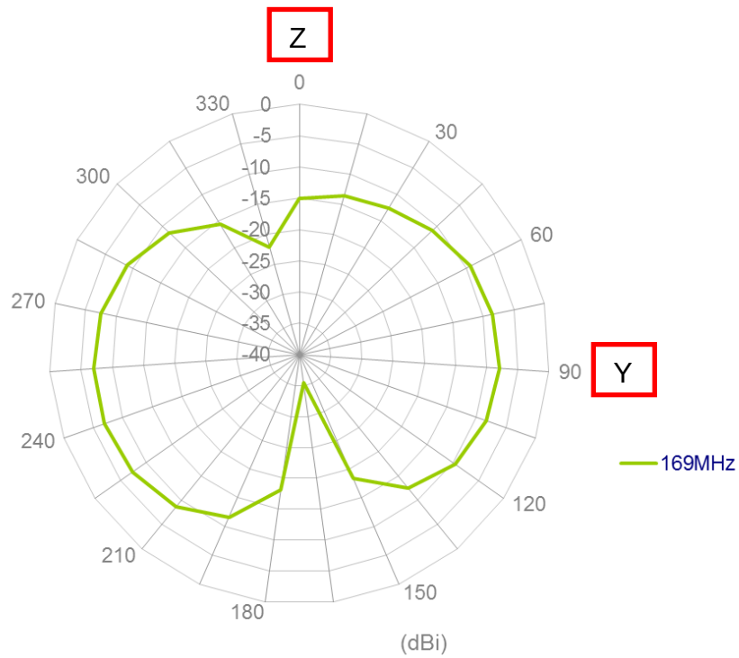
YZ-Plane
