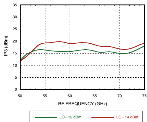
Input IP3, LO= 49 GHz, USB
