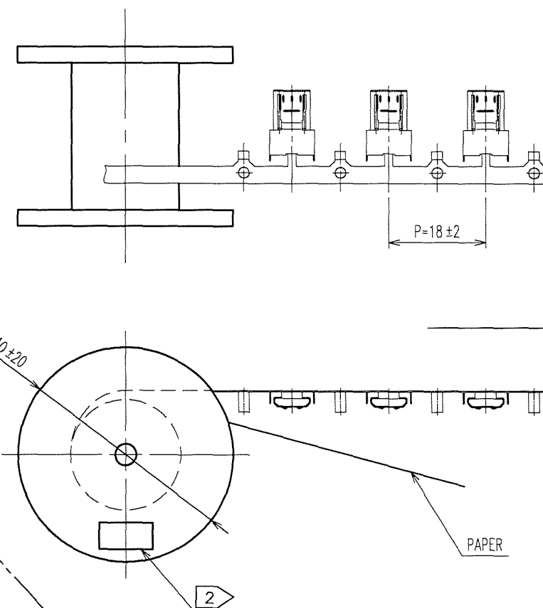
1 Fig-1 REELING(FREE)
