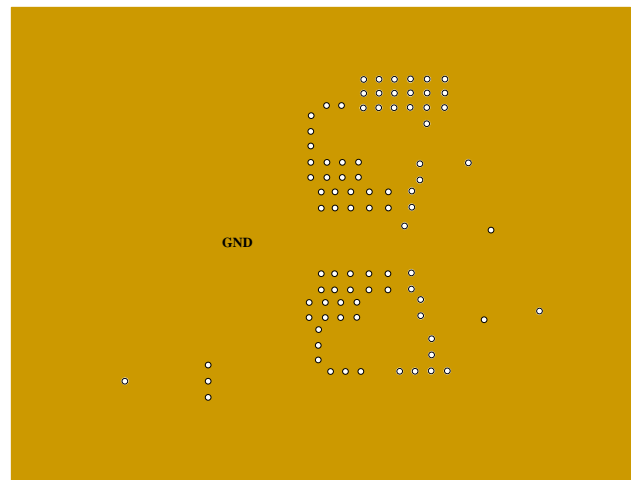
Inner1 Layer
