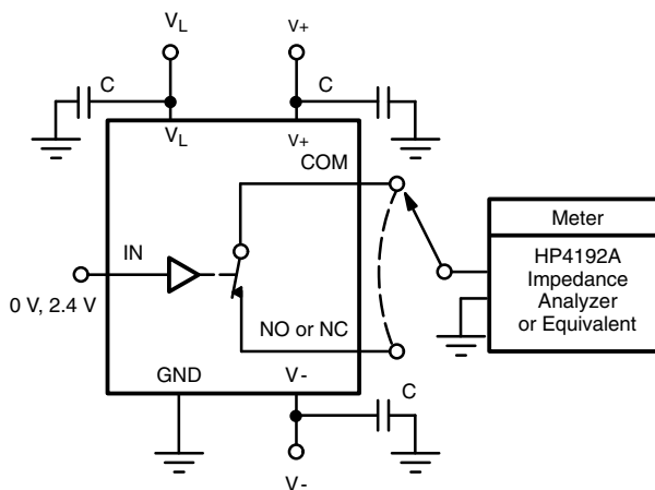
Fig. 7 - Source/Drain Capacitances
