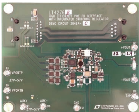
Top Side
