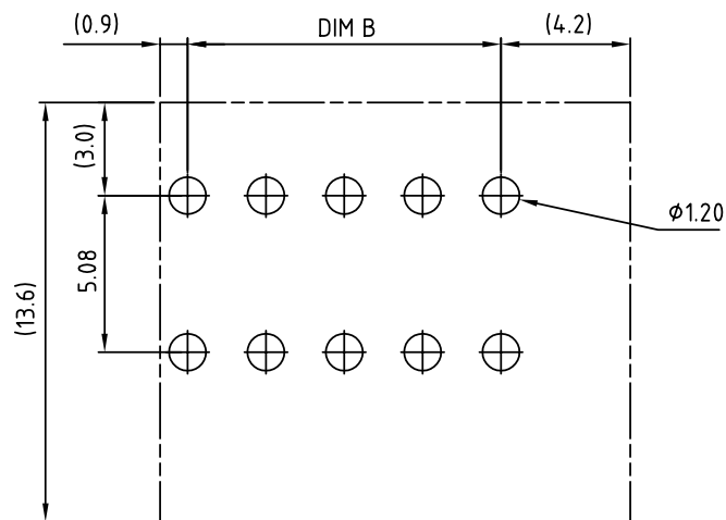
P.C.B. LAYOUT
