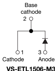
2L TO-220AC
