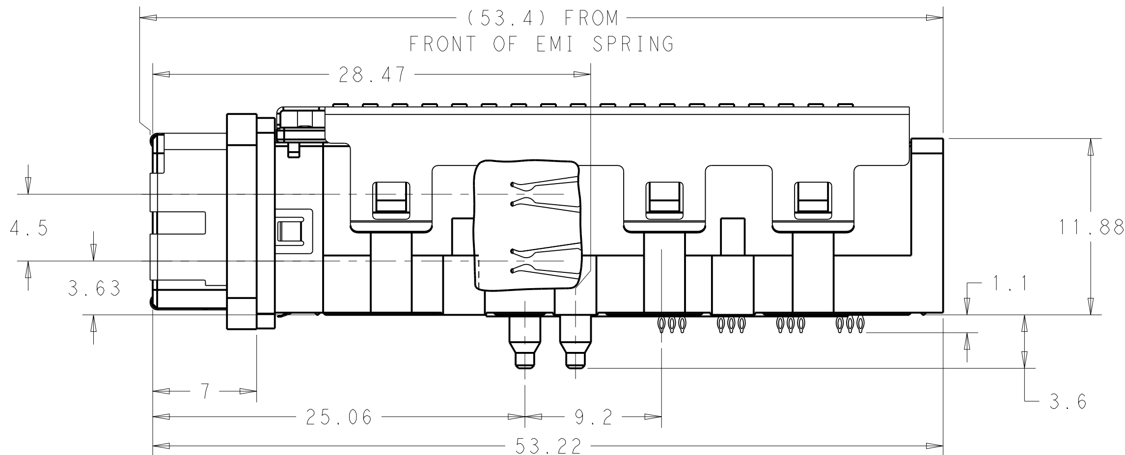
2149157-1 SCALE 4:1
