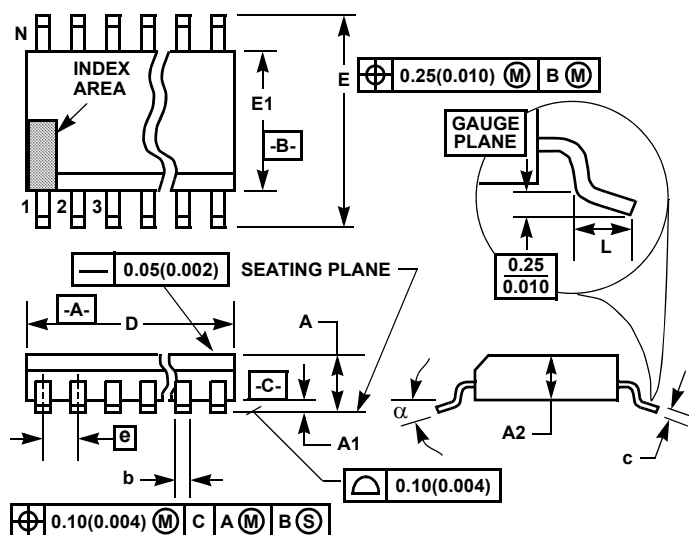
SYMBOL INCHES MILLIMETERS NOTES MIN MAX MIN MAX A - 0.043 - 1.10 - A1 0.002 0.006 0.05 0.15 - A2 0.033 0.037 0.85 0.95 - b 0.0075 0.012 0.19 0.30 9 c 0.0035 0.008 0.09 0.20 - D 0.193 0.201 4.90 5.10 3 E1 0.169 0.177 4.30 4.50 4 e 0.026 BSC 0.65 BSC - E 0.246 0.256 6.25 6.50 - L 0.020 0.028 0.50 0.70 6 N 16 16 7 \alpha 0° 8° 0° 8° -
