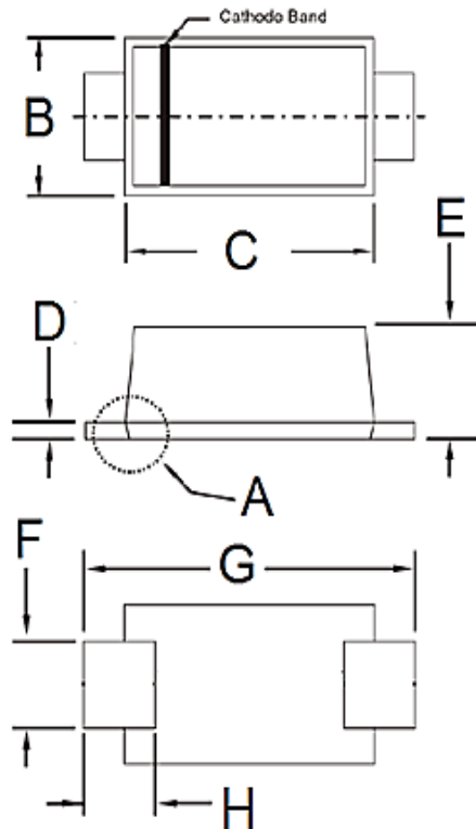
SOD-123W
