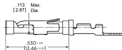
Socket
