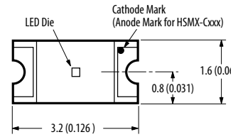
HSMx-C150
