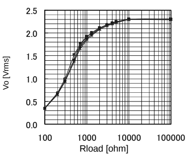
Fig.18 Rload vs Vo
