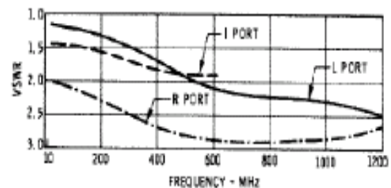
VSWR
