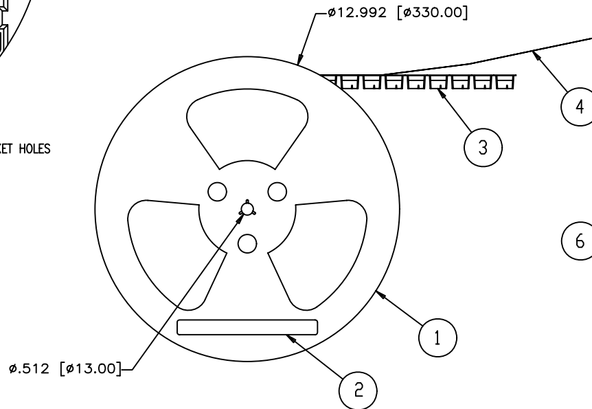
U77-A111X-XX0R SHOWN
