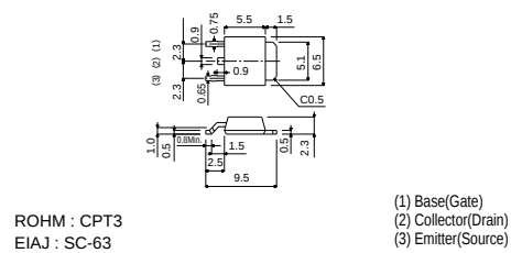
2SD1918
