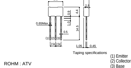
2SD1857A
