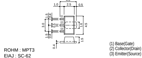
2SD2211
