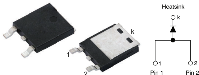
SlimDPAK (TO-252AE)
