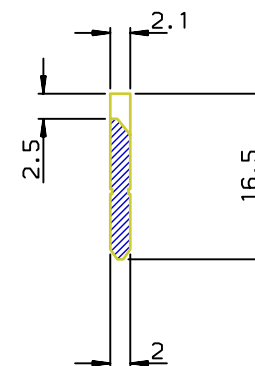
COUPE AA
