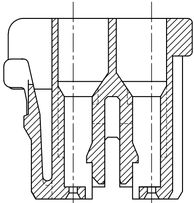
SECT A-A
