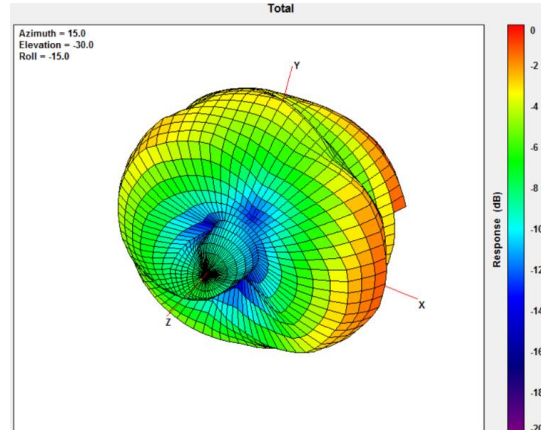
960MHz
