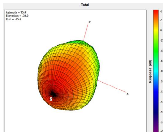
2170MHz
