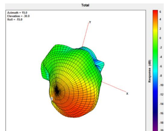
2690MHz
