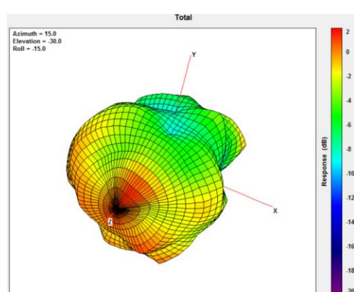
3500MHz
