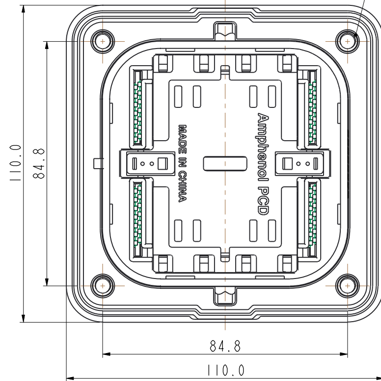
MSD RECEPTACLE
