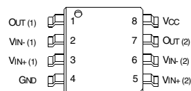
TS482IST - MiniSO-8
