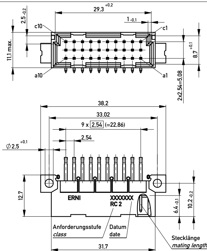
Bestückungsplan / contact layout
