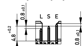
Stecklänge / mating length
