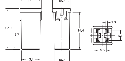
Dimensions JCASE®
