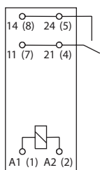
SPST (1NO)
