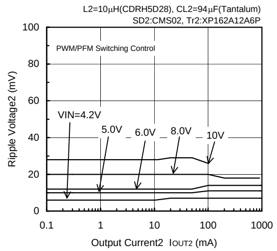
FOSC=500kHz, VOUT2=3.3V
