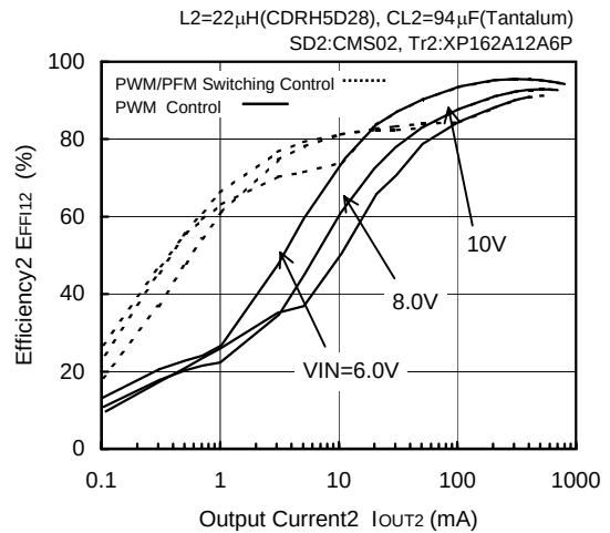
FOSC=300kHz, VOUT2=5.0V
