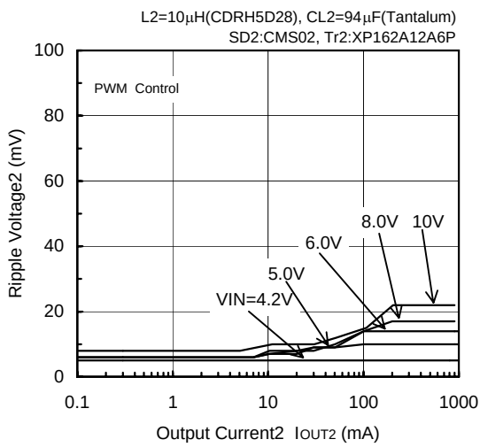
FOSC=500kHz, VOUT2=5.0V
