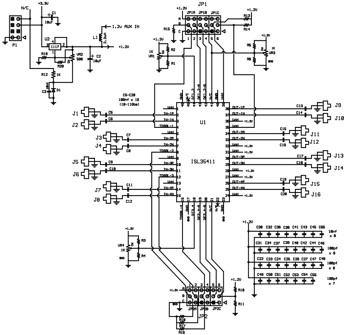
FIGURE 7. ISL35411DRZ-EVALZ SCHEMATIC
