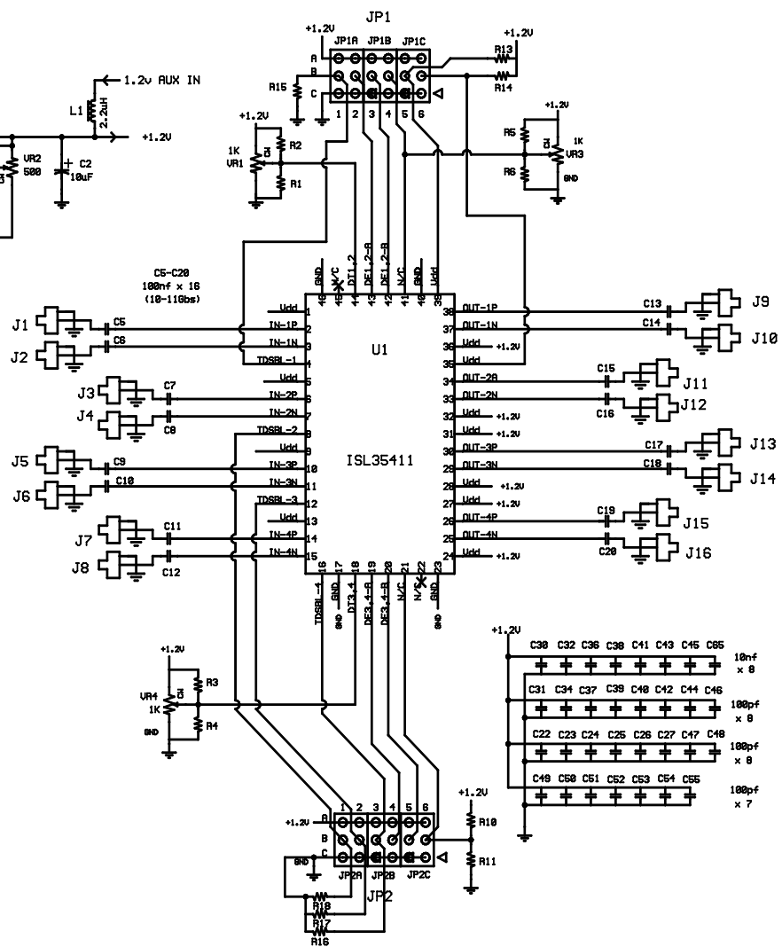
FIGURE 7. ISL35411DRZ-EVALZ SCHEMATIC
