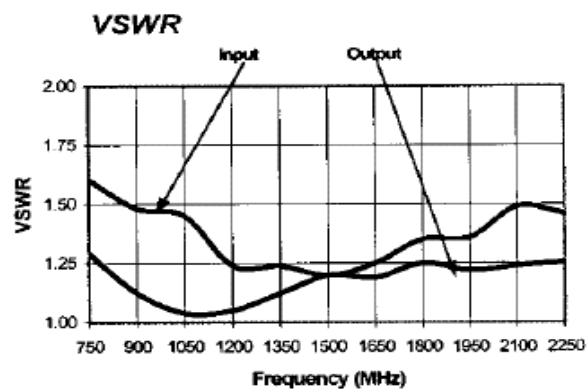
VSWR
