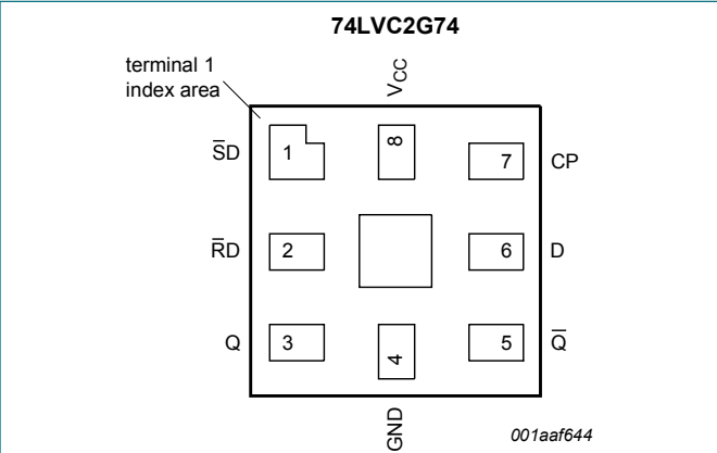
Fig. 6. Pin configuration SOT902-2 (XQFN8)
