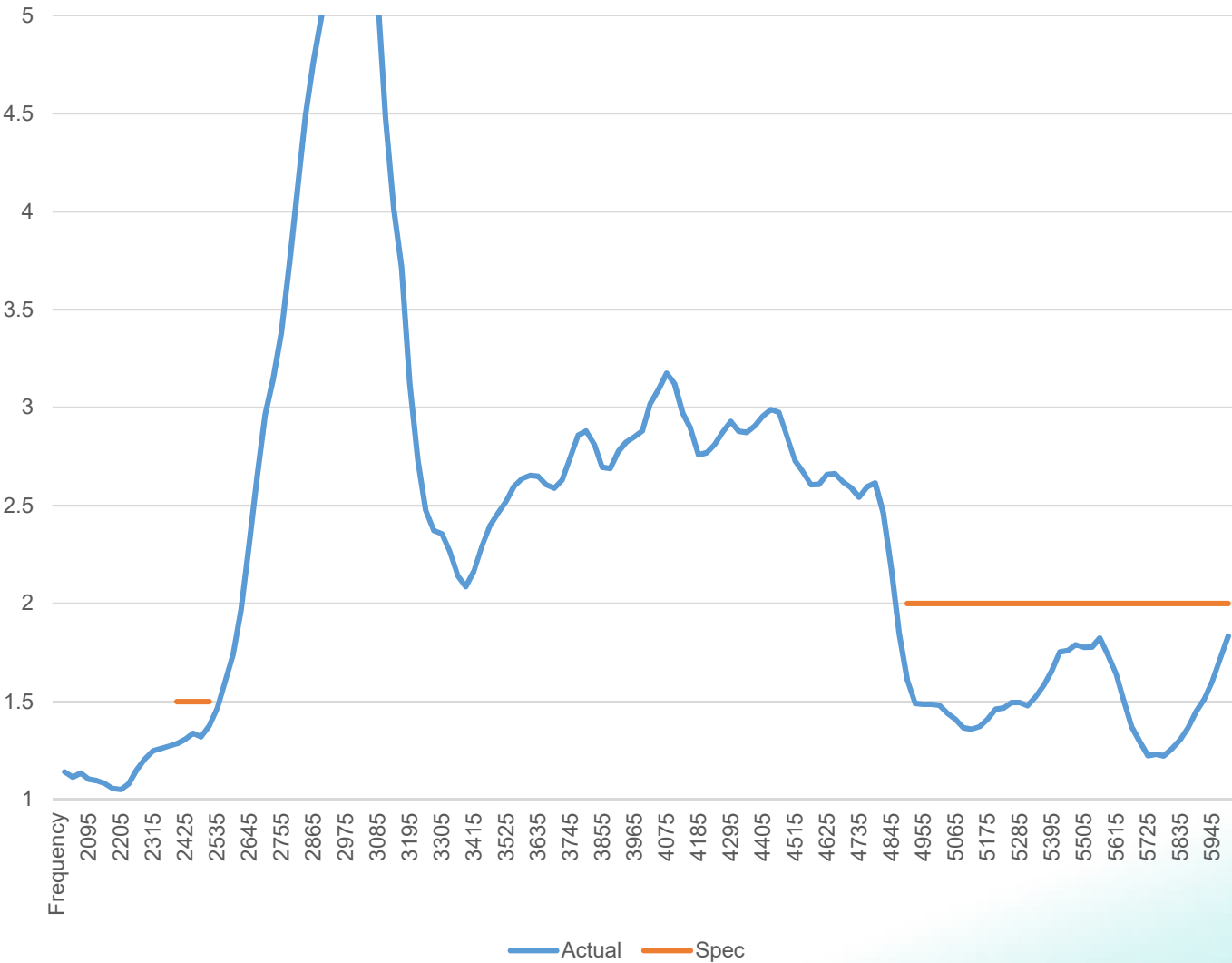
ICEFINWDMN VSWR
